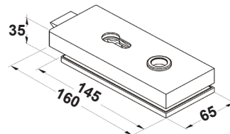
PL002S Beltéri ajtózárral, cylinderbetétes, szálcsiszolt, polír, eloxált alumínium
