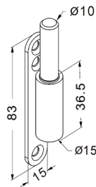
4006 Ajtócsap, tokra szerelhető háromrészes pánthoz, kérhető DIN tokhoz is (FH410C), acél
