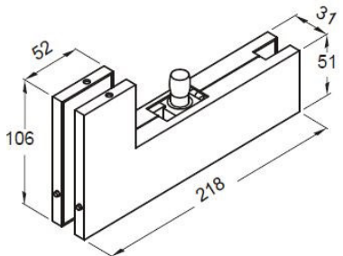
GF410L Ajtó felsőforgáspont ellendarab, jobbos / balos, oldal-, felüvilágító- és bordarögzítéssel, szálcsiszolt, eloxált alumínium
