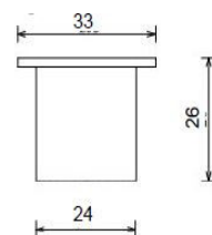
8825 Sarokzár ellendarab, zárhüvely, szálcsiszolt
