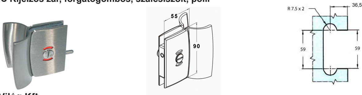
ILH700C Kijelzős zár, forgatógombos, szálcsiszolt, polír
