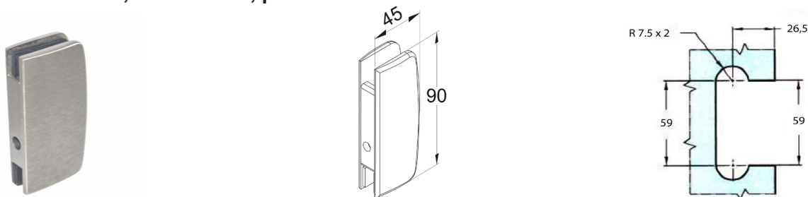
IL702C Zár ellendarab, szálcsiszolt, polír
