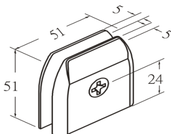
GC701G Fal-üveg, fix megfogó, szálcsiszolt, polír
