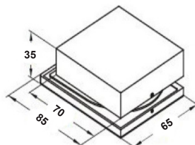
PL018R Beltéri ajtózárral ellendár rövid, szálcsiszolt
