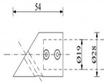
SB045 Indító, szálcsiszolt, polír
