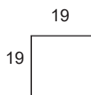
SB011 19 mm átmérőjű cső, SS011 19x19 mm zártszelvény, 2000 mm hosszban, szálcsiszolt, polír
