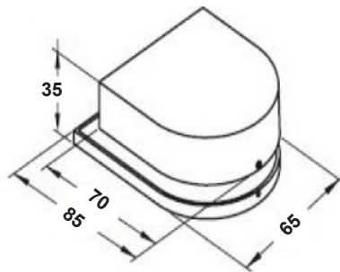
PL018S Beltéri ajtózárral ellendár rövid, szálcsiszolt
