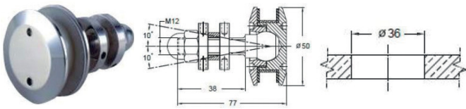
CAP30 Átmenőfuratos, menetes pontmegfogó, menetes távtartóval, szálcsiszolt
