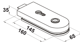
PL002S Beltéri ajtózárral, cylinderbetétes, szálcsiszolt, polír, eloxált alumínium
