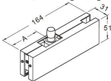
GF400 Ajtó felsőforgáspont ellendarab, oldal- és felüvilágító rögzítéssel, szálcsiszolt, eloxált alumínium
