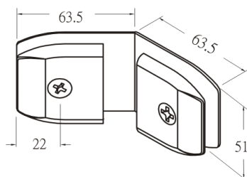
GC706G 90° Talpas, fal-üveg, fix megfogó, szálcsiszolt, polír
