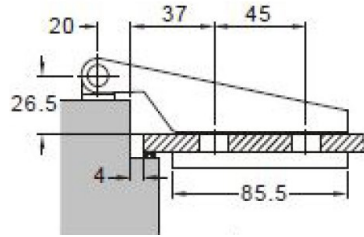
FH401G Tokba való, talpas felnyíló ajtópánt, szálcsiszolt (45kg / 2 pánt)
