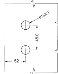
FH411C Tokba való, talpas felnyíló ajtópánt, szálcsiszolt (45kg / 2 pánt)
