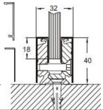
8816 Ajtó alsó forgáspont ellendarab (74-75AX), szálcsiszolt
