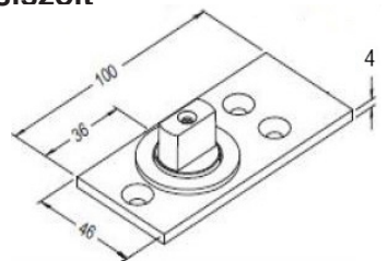
8825 Sarokzár ellendarab, zárhüvely, szálcsiszolt
