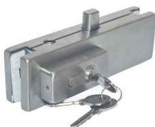
GL200N Középzár, szálcsiszolt, eloxált alumínium
