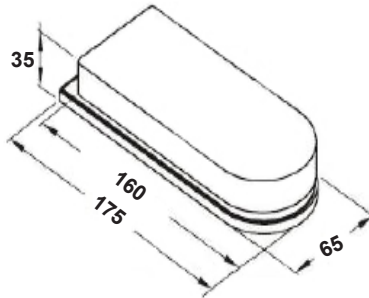
PL008G Beltéri ajtózárral ellendár, szálcsiszolt
