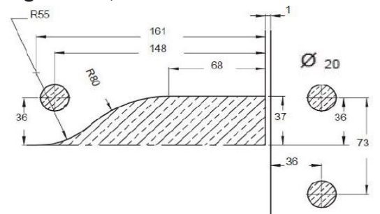
GF410L Ajtó felsőforgáspont ellendarab, jobbos / balos, oldal-, felüvilágító- és bordarögzítéssel, szálcsiszolt, eloxált alumínium
