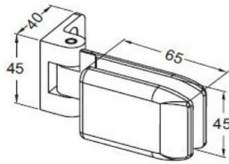
FH103G Felnyíló ajtópánt, szálcsiszolt, polír (36kg / 2pánt)
