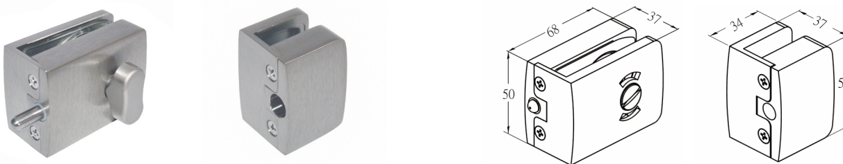
IL702C Zár ellendarab, szálcsiszolt, polír
