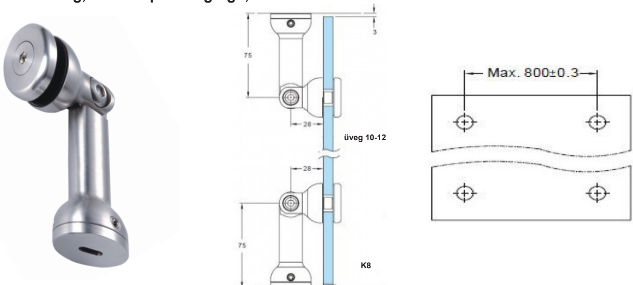
GC03075F Fal-üveg, csuklós pontmegfogó, szálcsiszolt
