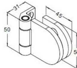
FH803R Dupla furatos üveg-üveg szaunapánt, szálcsiszolt, polír (28kg / 2 pánt)
