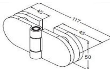
FH803R Dupla furatos üveg-üveg szaunapánt, szálcsiszolt, polír (28kg / 2 pánt)
