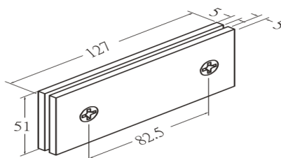
GC703S 180°-os üveg-üveg, fix megfogó, szálcsiszolt, polír
