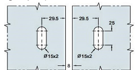
FH803R Dupla furatos üveg-üveg szaunapánt, szálcsiszolt, polír (28kg / 2 pánt)
