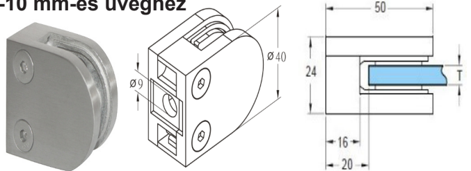
BC050 Pontmegfogó, furat nélkül, szálcsiszolt 6-10 mm-es üveghez
