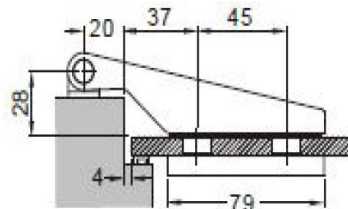
FH400N Felnyíló ajtópánt, szálcsiszolt, polírozott (40kg / 2 pánt)
