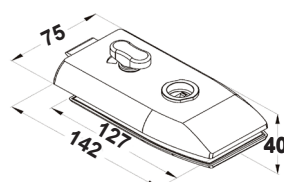
WLI012G Beltéri kijelzős ajtózárral, forgatógombos, cylinderbetétes, szálcsiszolt
