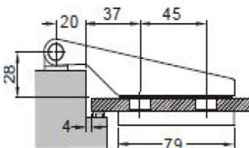
FH400G Felnyíló ajtópánt, szálcsiszolt (40kg / 2 pánt)
