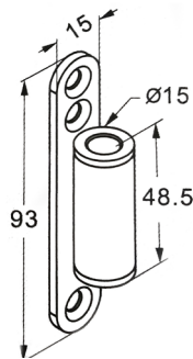
4006 Ajtócsap, tokra szerelhető háromrészes pánthoz, kérhető DIN tokhoz is (FH410C), acél
