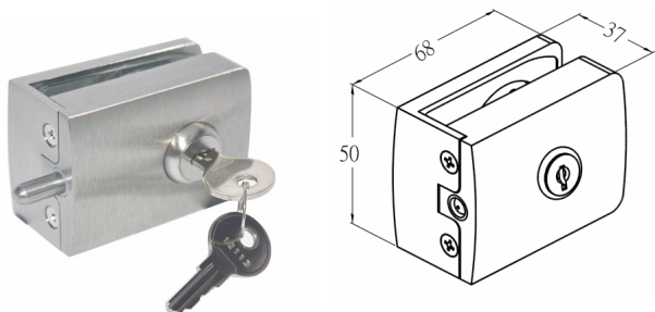
IL600C Ráhúzható, kijelzős zár forgatógombos, szálcsiszolt
