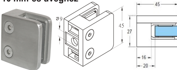
GC03075F Fal-üveg, csuklós pontmegfogó, szálcsiszolt
