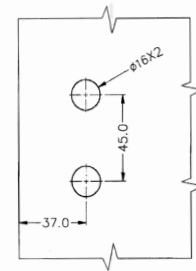
FH410C Háromrészes, felnyíló ajtópánt, szálcsiszolt (45kg / 2 pánt)
