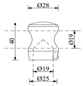
SB007 Állítható rúdösszekötő, szálcsiszolt, polír
