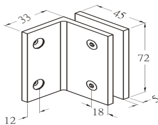
GC701G Fal-üveg, fix megfogó, szálcsiszolt, polír
