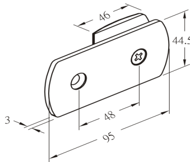
GC807C 90° Talpas, fal-üveg, fix megfogó, szálcsiszolt, polír
