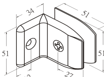
GC706G 90° Talpas, fal-üveg, fix megfogó, szálcsiszolt, polír
