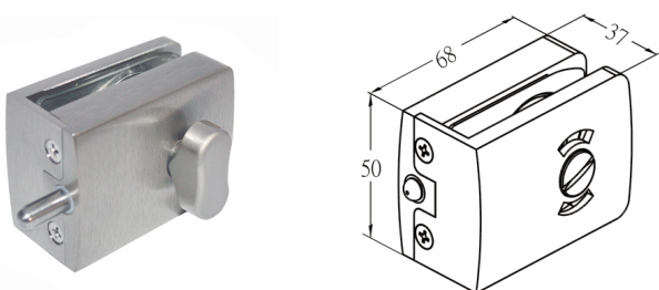
IL600C Ráhúzható, kijelzős zár forgatógombos, szálcsiszolt
