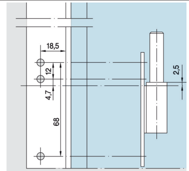
4006 Ajtócsap, tokra szerelhető háromrészes pánthoz, kérhető DIN tokhoz is (FH410C), acél
