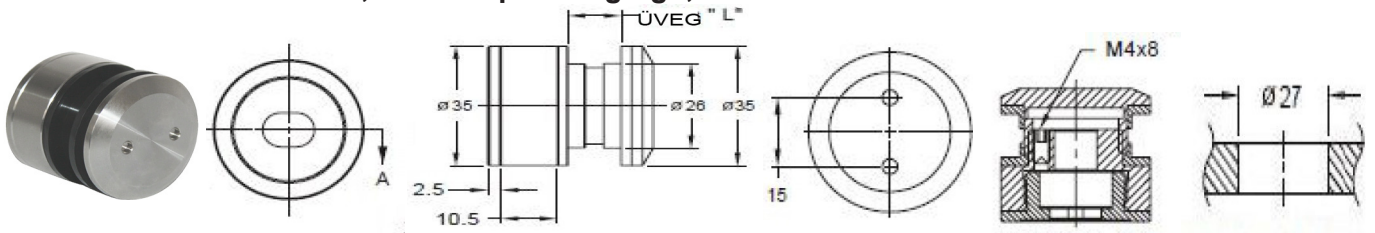
SF0010 Átmenőfuratos pontmegfogó fej, szálcsiszolt
