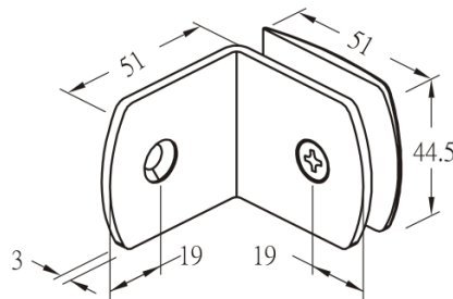
GC807C 90° Talpas, fal-üveg, fix megfogó, szálcsiszolt, polír
