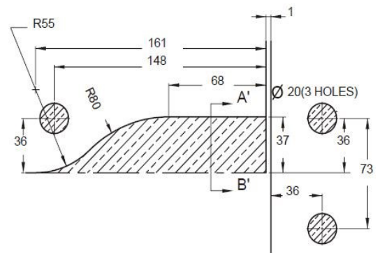
GF410L Ajtó felsőforgáspont ellendarab, jobbos / balos, oldal-, felüvilágító- és bordarögzítéssel, szálcsiszolt, eloxált alumínium
