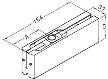
GF300 Ajtó felsőforgáspont ellendarab, felüvilágító rögzítéssel, szálcsiszolt, eloxált alumínium
