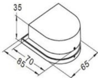
PL018G Beltéri ajtózárral ellendárab rövid, szálcsiszolt
