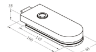
PL006S Beltéri ajtózárral, csak kilincses, szálcsiszolt, polír, eloxált alumínium
