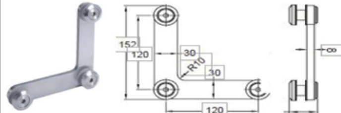
PD700F Oldal és felülvilágító rögzítéssel szálcsiszolt
