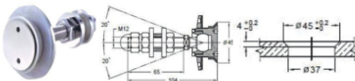
SF13812AF Átmenőfuratos, állítható pontmegfogó, szálcsiszolt
