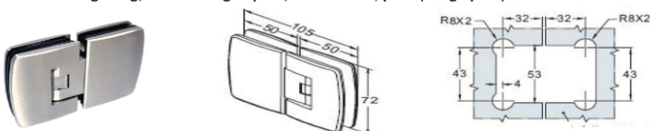
AH404C 90° Üveg-üveg, állítható rugós pánt, szálcsiszolt, polír (28kg/2pánt)
