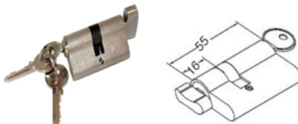
TC02 30/30 forgatógombos zárbetét, 3 kulcsos
