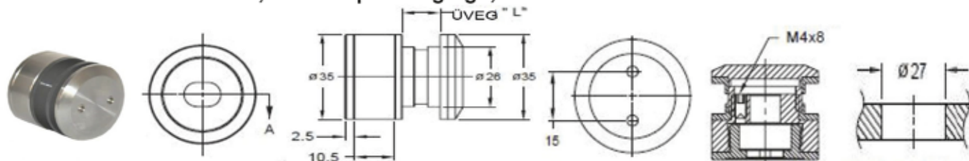
CAP30 Átmenőfuratos pontmegfogó, kérésre egyedi távtartóval, szálcsiszolt
