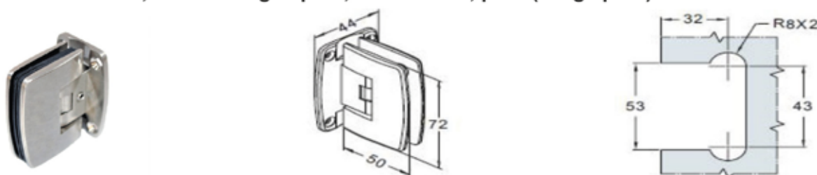
AH401C Szimmetrikus, állítható rugós pánt, szálcsiszolt, polír (28kg/2pánt)
