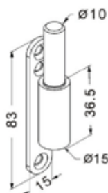
4006 háromrészes pánthoz, tokra szerelhető ajtócsap, kérhető DIN tokhoz való is (FH410C-hez), acél
