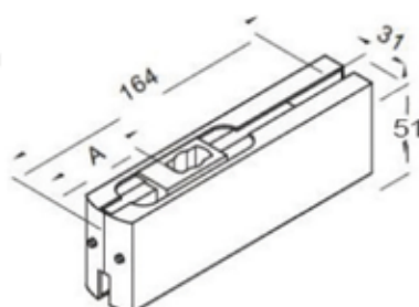
GF100 Ajtó alsóforgáspont, szálcsiszolt, eloxált alumínium
