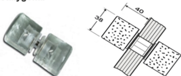
Mágneses rögzítő, szauna ajtóhoz
