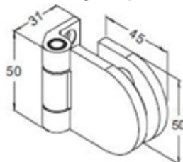
FH803R Üveg-üveg, dupla furatos pánt, szálcsiszolt, polír (28kg / 2 pánt)
