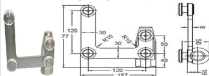
PD500F Ajtó felső forgáspont ellendarab, szálcsiszolt
