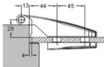
FH401G Tokba való, felnyíló ajtópánt, szálcsiszolt (45kg / 2 pánt)
