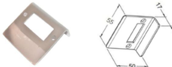
PL07C Falra szerelhető zárlemez, szálcsiszolt
