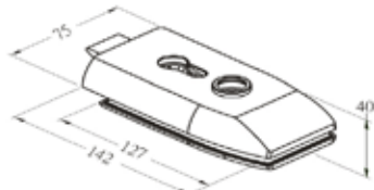
PL012G Beltéri ajtózárral, cylinderbetétes, szálcsiszolt
