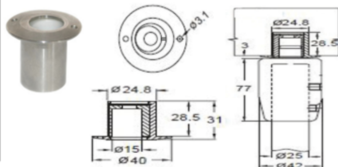
PD700F Oldal és felülvilágító rögzítéssel szálcsiszolt
