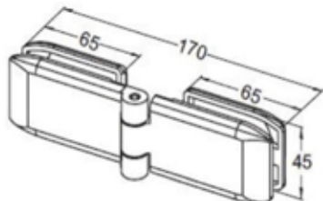
FH400C Felnyíló ajtópánt, csak eloxált alumínium (40kg / 2 pánt)
