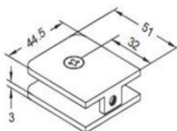
GC801C Fal-üveg, fix megfogó, szálcsiszolt, polír
