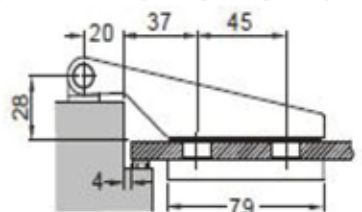
FH400N Felnyíló ajtópánt, szálcsiszolt, polírozott (40kg / 2 pánt)
