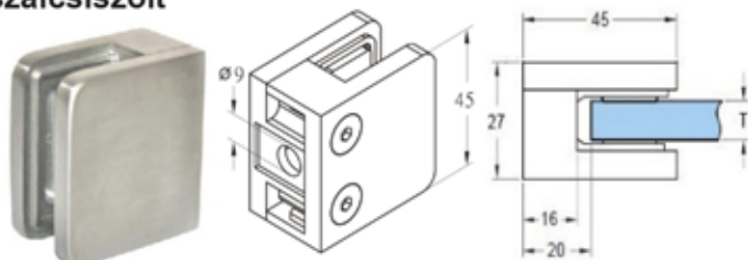
GC03075F Fal-üveg, csuklós pontmegfogó, szálcsiszolt
