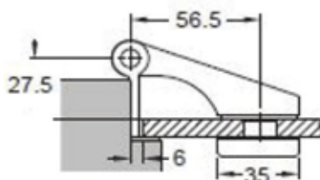
FH801R Felnyíló ajtópánt, dupla furatos szaunapánt, szálcsiszolt, polír (28kg / 2 pánt)
