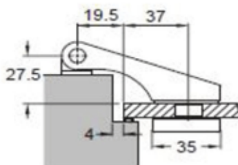
FH411C Tokba való, felnyíló ajtópánt, szálcsiszolt (45kg / 2 pánt)
