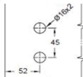
FH801R Felnyíló ajtópánt, dupla furatos szaunapánt, szálcsiszolt, polír (28kg / 2 pánt)
