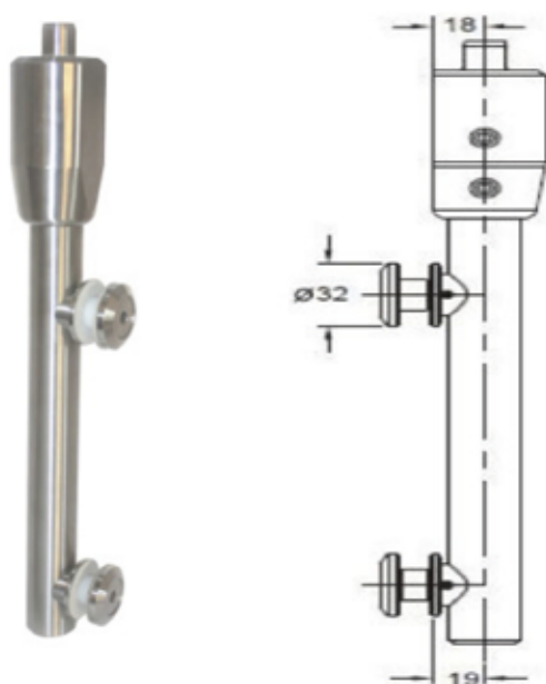
PD200F Ajtó felső forgáspont, szálcsiszolt
