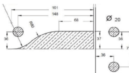
GF410L Ajtó felsőforgáspont ellendarab, jobbos / balos, oldal-, felülvilágító és bordarögzítéssel, szálcsiszolt, eloxált alumínium
