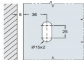
FH801R Felnyíló ajtópánt, dupla furatos szaunapánt, szálcsiszolt, polír (28kg / 2 pánt)
