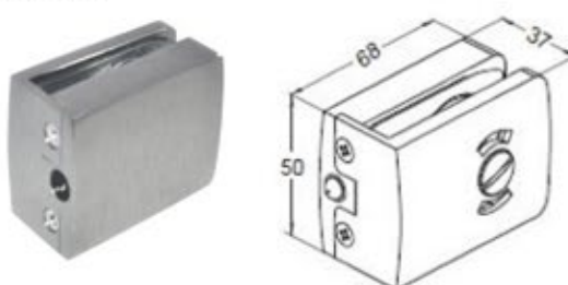
IL601C Ráhúzható zár ellendarab, szálcsiszolt
