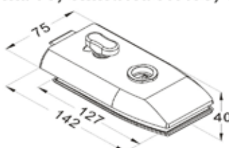
WLI012G Beltéri kijelzős ajtózárral, forgatógombos, cylinderbetétes, szálcsiszolt
