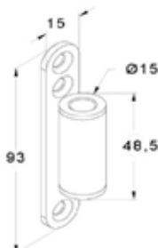
4006 háromrészes pánthoz, tokra szerelhető ajtócsap, kérhető DIN tokhoz való is (FH410C-hez), acél
