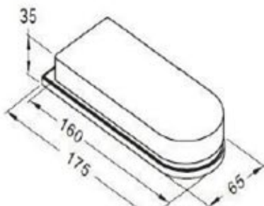
PL008G Beltéri ajtózárral ellendárab, szálcsiszolt
