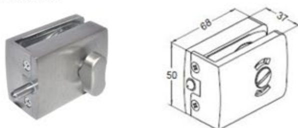
IL600C Ráhúzható, kijelzős zár, szálcsiszolt
