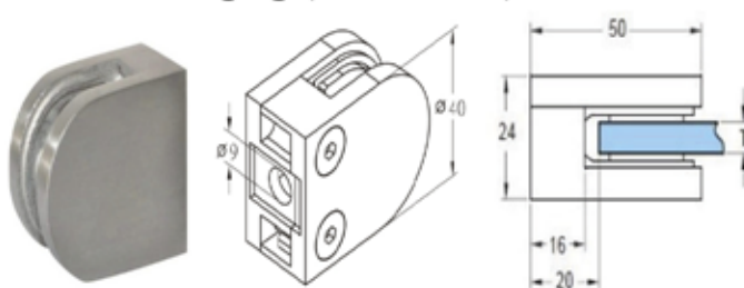
BC050 Pontmegfogó, furat nélkül, szálcsiszolt
