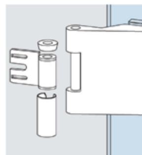
4006 háromrészes pánthoz, tokra szerelhető ajtócsap, kérhető DIN tokhoz való is (FH410C-hez), acél
