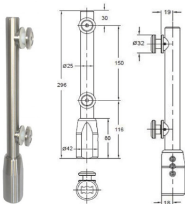
PD100F Alsó forgáspont, szálcsiszolt
