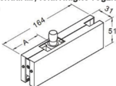
GF400 Ajtó felsőforgáspont ellendarab, oldal- és felülvilágító rögzítéssel, szálcsiszolt, eloxált alumínium
