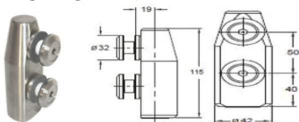
PD200F Ajtó felső forgáspont, szálcsiszolt
