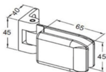
FH102G Felnyíló ajtópánt, szálcsiszolt, polír (36kg / 2pánt)
