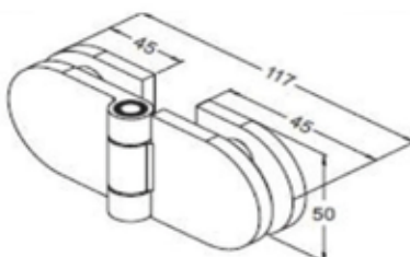
FH803R Üveg-üveg, dupla furatos pánt, szálcsiszolt, polír (28kg / 2 pánt)
