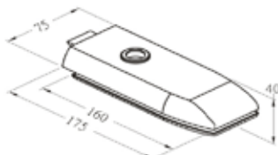
PL002R Beltéri ajtózárral, cylinderbetétes, szálcsiszolt
