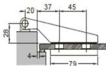
FH400N Felnyíló ajtópánt, szálcsiszolt, polírozott (40kg / 2 pánt)
