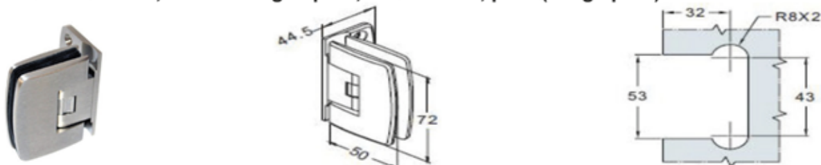
AH401C Szimmetrikus, állítható rugós pánt, szálcsiszolt, polír (28kg/2pánt)
