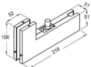
GF410L Ajtó felsőforgáspont ellendarab, jobbos / balos, oldal-, felülvilágító és bordarögzítéssel, szálcsiszolt, eloxált alumínium
