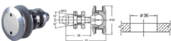
SF010 Átmenőfuratos pontmegfogó fej, szálcsiszolt
