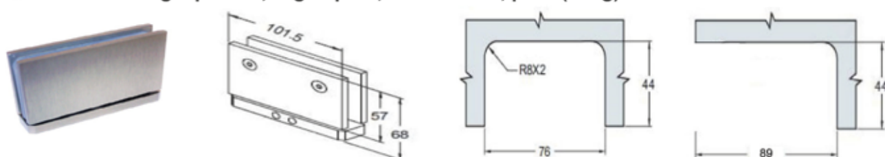
AH503S Forgáspontos rugós pánt, felülvilágító rögzítéssel, szálcsiszolt (60kg)
