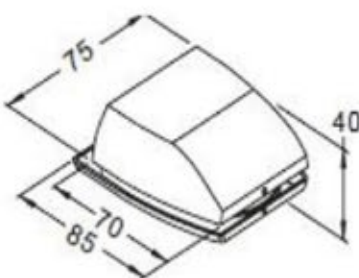
PL018R Beltéri ajtózárral ellendárab rövid, szálcsiszolt
