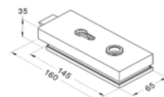
PL002S Beltéri ajtózárral, cylinderbetétes, szálcsiszolt, polír, eloxált alumínium
