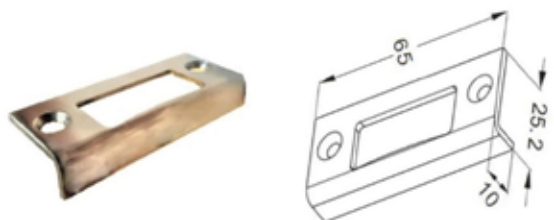
KP03 Tokra szerelhető zárlemez, szálcsiszolt
