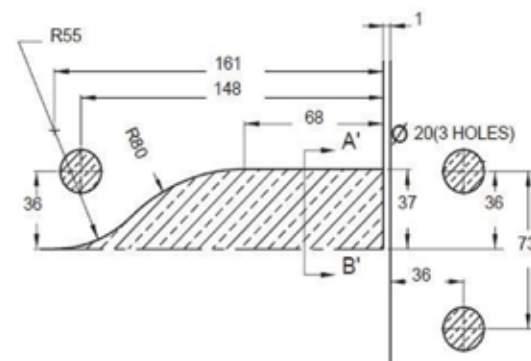
GF410L Ajtó felsőforgáspont ellendarab, jobbos / balos, oldal-, felülvilágító és bordarögzítéssel, szálcsiszolt, eloxált alumínium
