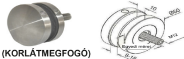
BC050 Pontmegfogó, furat nélkül, szálcsiszolt
