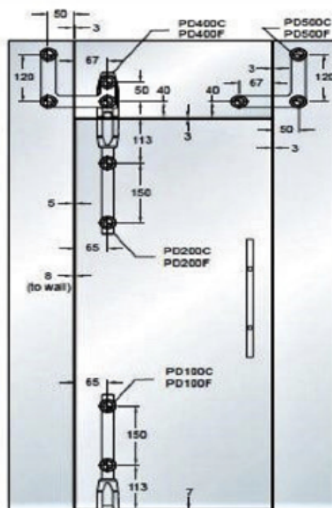
PD400F Ajtó felső forgáspont ellendarab, oldal és felülvilágító rögzítéssel, szálcsiszolt
